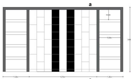
OSARIO PLANTA ÚNICA ESQ: 1:35
